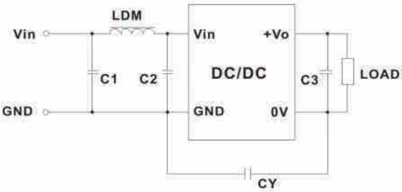
图7 EMC推荐电路
