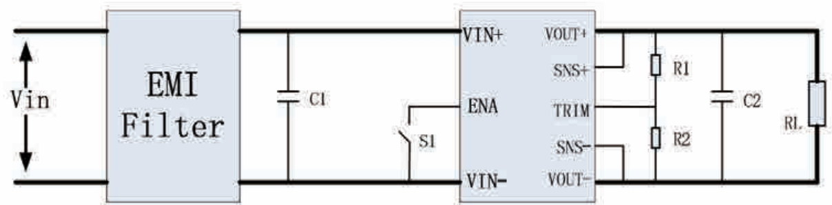
图2 典型应用电路
